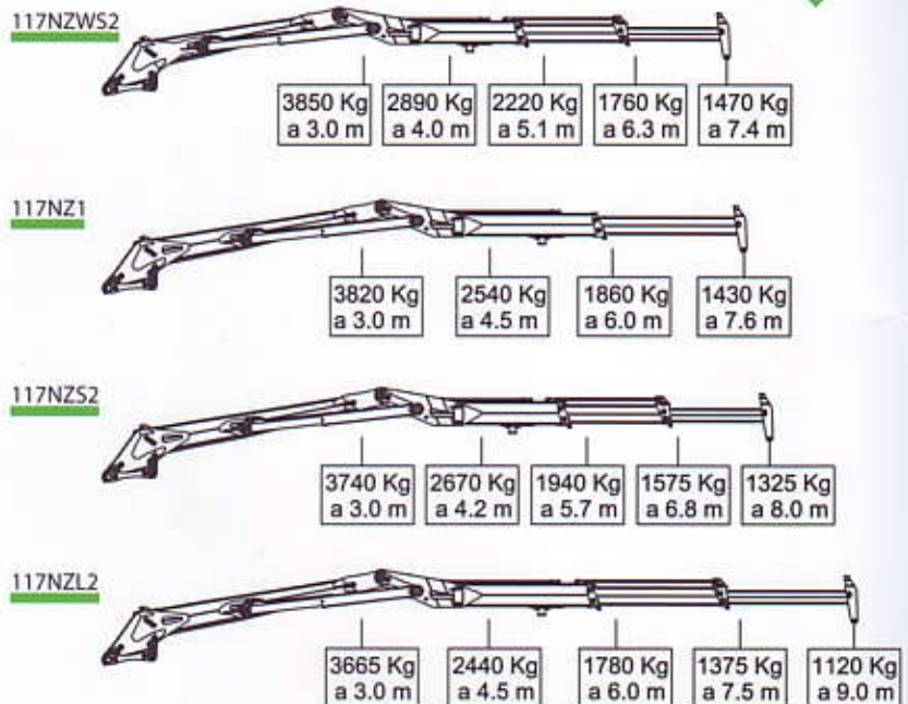
Diagrama de cargas / Diagrama de cargas Diagramme de charges / Load diagram
