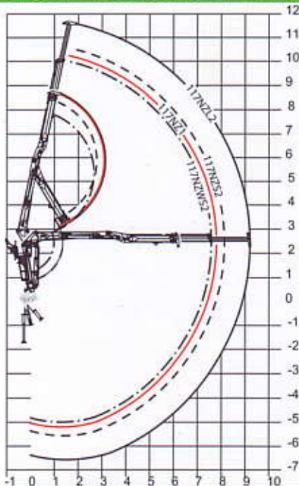
Diagrama de posiciones / Diagrama de posições Diagramme des positions / Positions diagram
